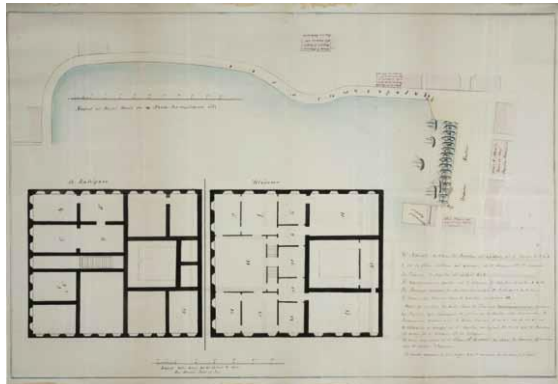
Τοπογραφικό σχέδιο [άγνωστης περιοχής] στο οποίο αποτυπώνονται οι θέσεις δημοσίων κτηρίων (Τελωνείου, Χαρτοφυλακείου, Υγειονομείου, Αστυνομίας) και κατοικιών, 1866. ΓΑΚ, αρχείο Υπουργείου Οικονομικών-Εθνικά Κτήματα
