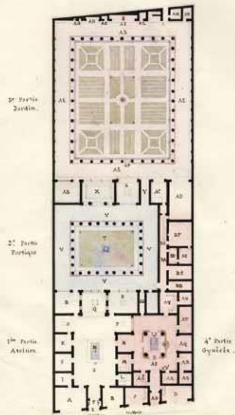
Plan. de la Maison du faune ou de la grande mosaïque, à Pompéïe.
