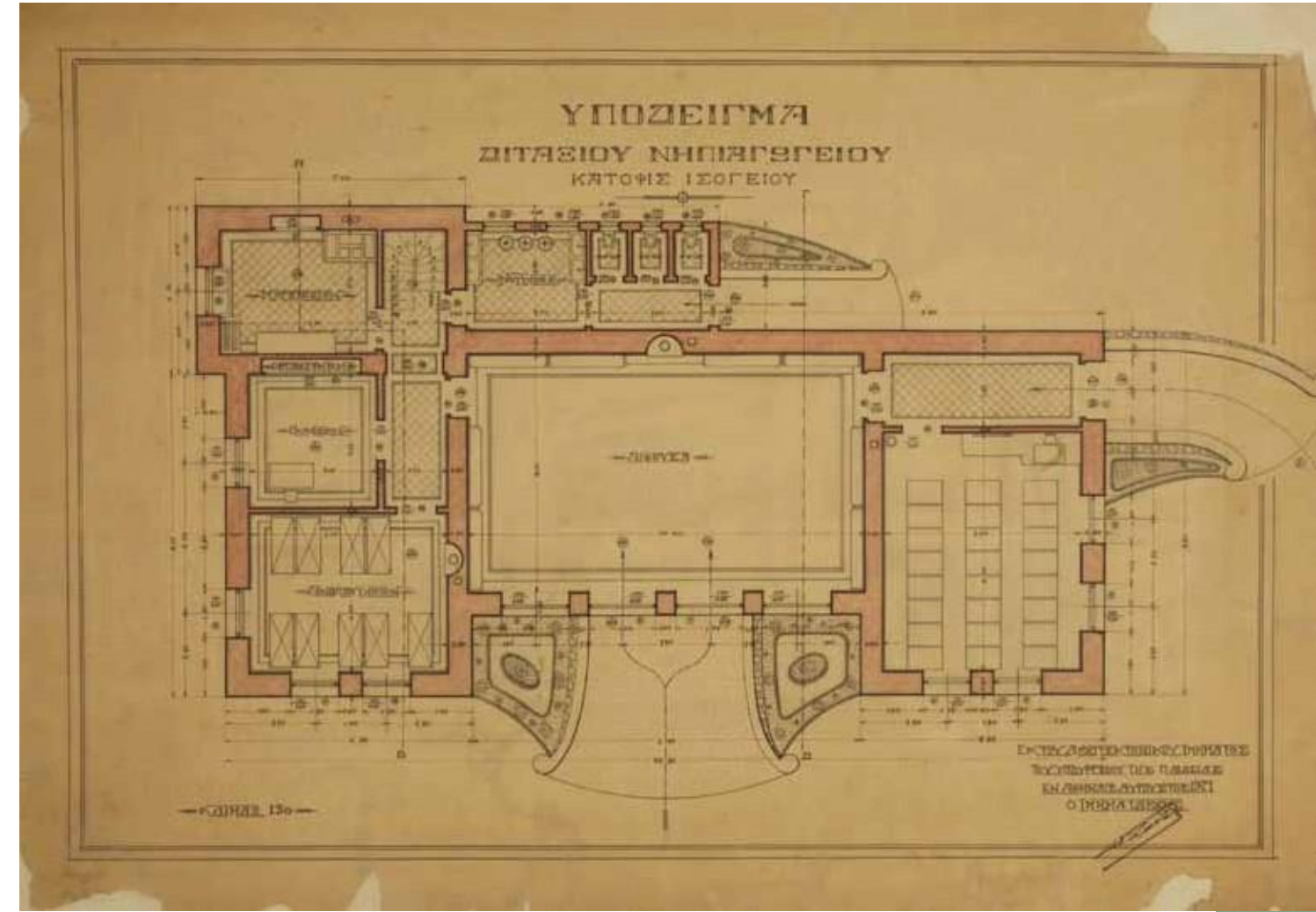
Υπόδειγμα διτάξιου Νηπιαγωγείου. Χρονολογία θεώρησης: 1921. ΓΑΚ, αρχείο Διεύθυνσης Τεχνικών Υπηρεσιών Υπουργείου Παιδείας & Θρησκευμάτων
