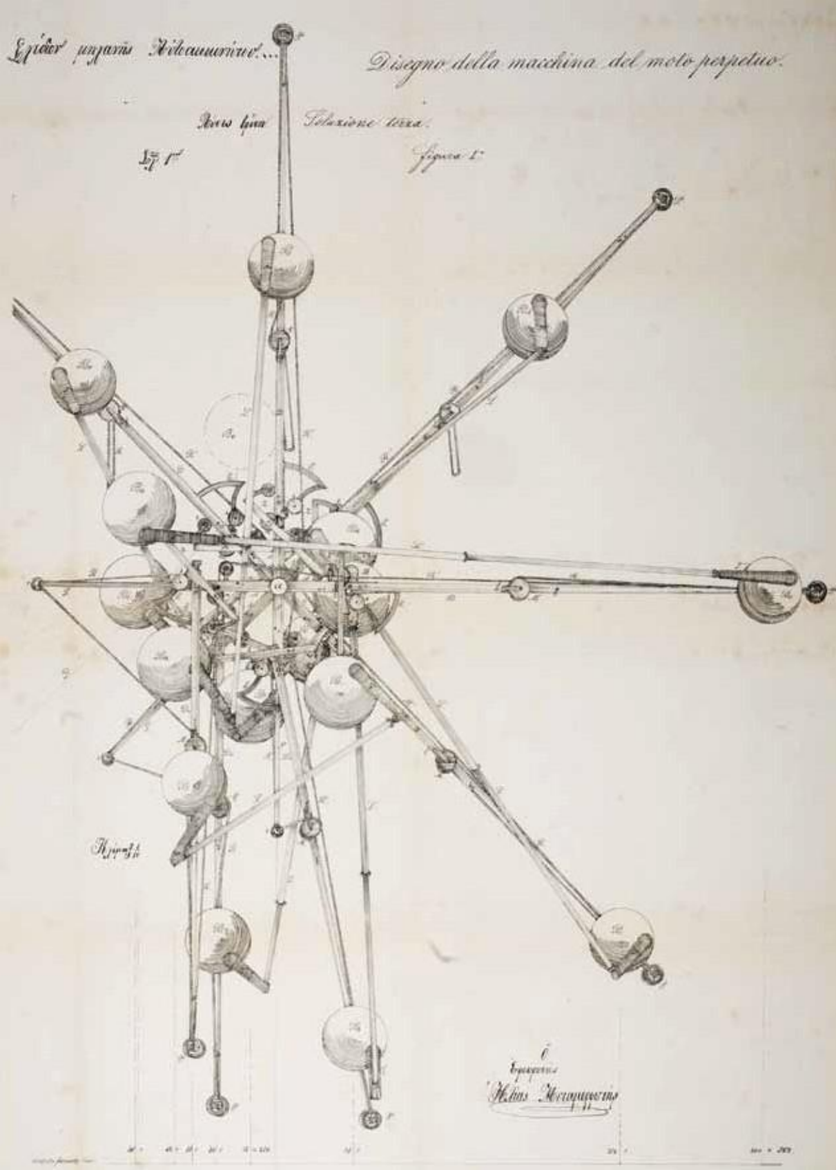
Σχέδιο κατασκευής μηχανής αυτοακίνητου το οποίο κατατέθηκε προς το Υπουργικό Συμβούλιο ως επισυναπτόμενο αίτησης για τη χορήγηση προνομίου εφευρέσεως. Τεργέστη, 12/24 Οκτωβρίου 1873. ΓΑΚ, αρχείο Υπουργείου Εσωτερικών
