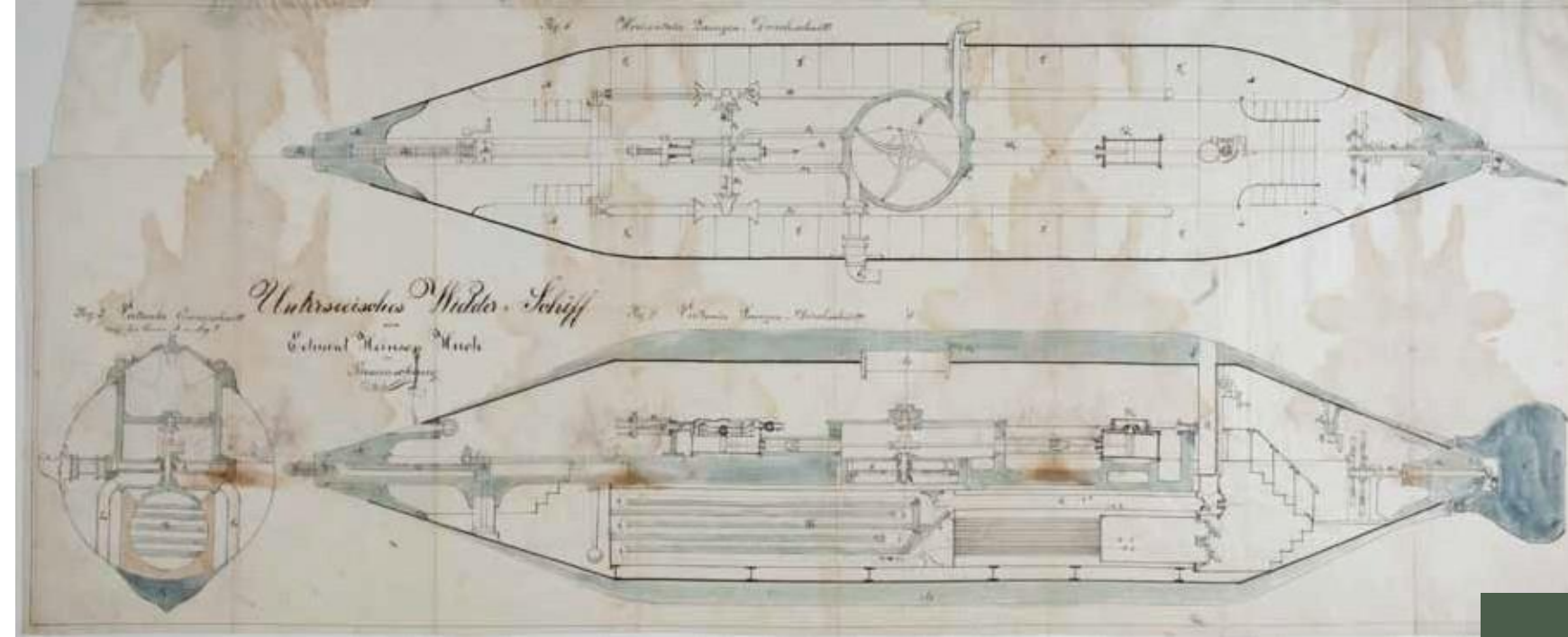
Σχέδιο υποβρυχίου, [19ος αι.] ΓΑΚ, αρχείο Υπουργείου Ναυτικών
