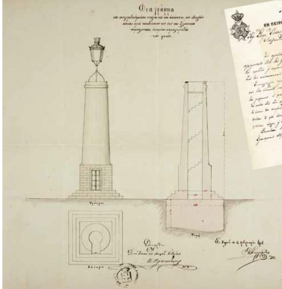
Οικονομική και τεχνική προσφορά του Μηχανουργείου «ΗΦΑΙΣΤΟΣ» σχετική με την κατασκευή στήλης για την τοποθέτηση φανού απέναντι από το Μπούρτζι. Επισυναπτάται σχέδιο. Πειραιάς, 7 Ιουλίου 1878.
